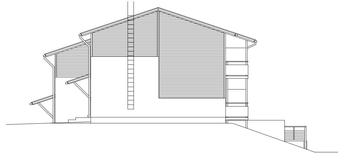
LUOTEESEEN
