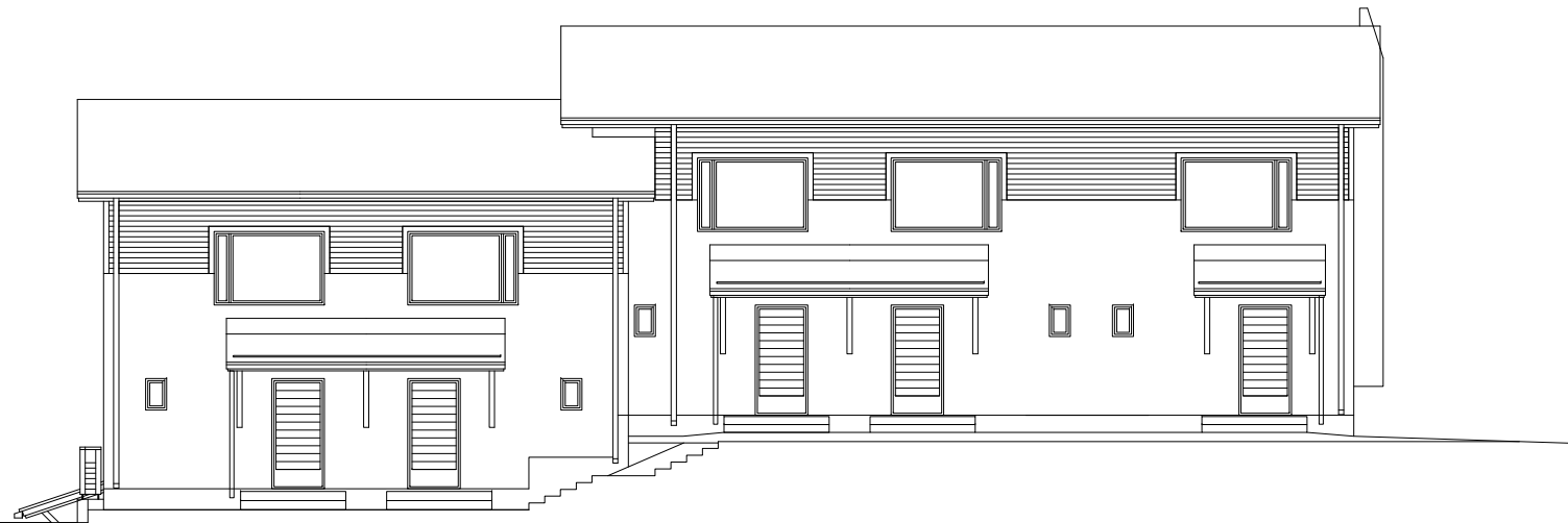
JULKISIVU KOILLISEEN
